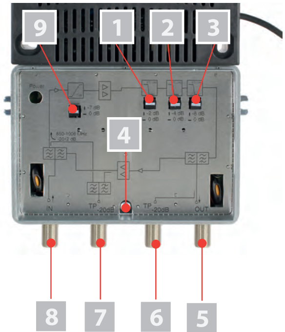
Bild 2: Verstärker HV 12 V3
