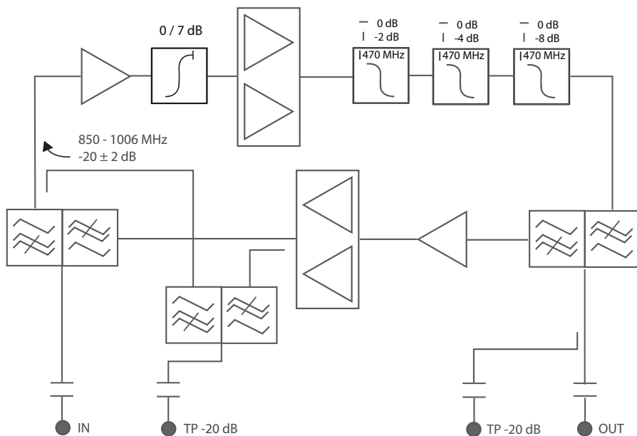
Blockschaltbild HV 12 V3
